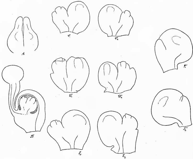
Fig. 1. A—E: Rigiostachys connaroides Loes. et Solldr., A Gynaeceum aus einer Blütenknospe, B Pistill einer entwickelten Blüte im medianen Längsschnitt, C—E Samenanlagen der Pistille C und E. F Samenanlage von Rigiostachys bracteata Planch. (Vergr. B 20 : 1, das übrige 36 : 1.)
